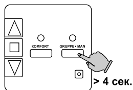
Групповой пульт Nero II 8413-50
